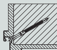
Toc de colț special montată în zidărie prin canalul garniturii de etanșare
