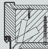
Ramă perimetrală montată în zidărie ancoră tip diblu pentru zid
