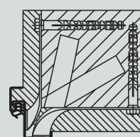
Toc de colț Montare în zidărie Ancoră tip diblu pentru zid
