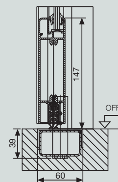
În livrarea standard fără opritor la partea inferioară, la cerere cu garnitură
