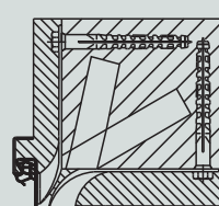
Toc de colț montată în zidărie ancoră tip diblu pentru zid
