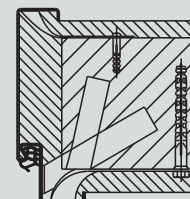
Ramă perimetrală Montare în zidărie Ancoră tip dublu pentru zid
